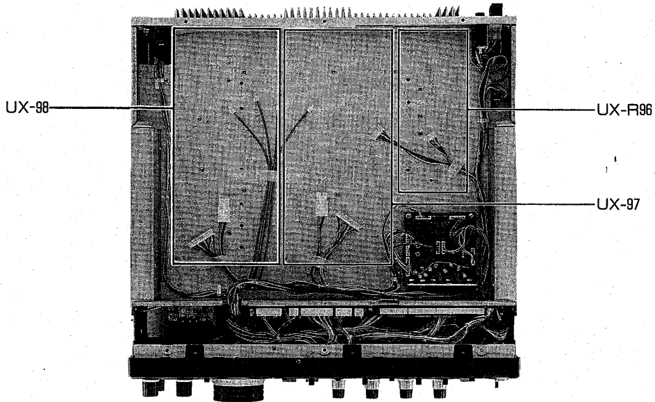
図3 下蓋内オプションユニット取り付け位置
