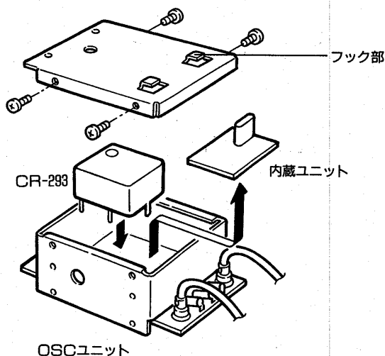
図12 CR-293の取り付け
