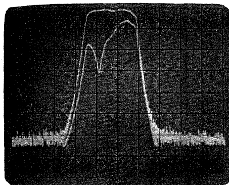
NOTCH回路の特性例
