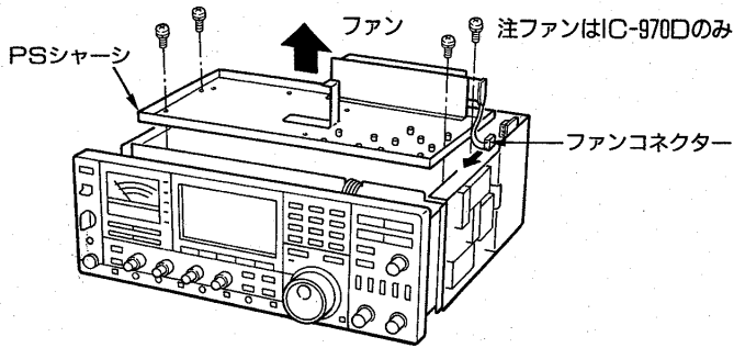
図14 PSシャーシの取り外し
