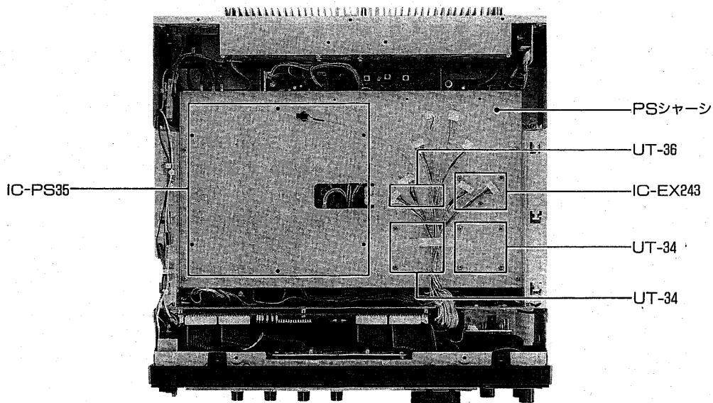
図2 上蓋内オプションユニット取り付け位置
